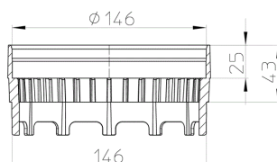
Schnitt A-A
