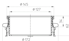
Schnitt A-A
